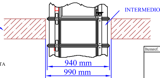
ESCALA 2:1 (CONFIGURACIÓN ATRAVESANDO SUELO)
