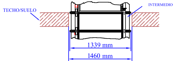
DETALLE "A" ESCALA 2:1 (CONFIGURACIÓN ATRAVESANDO SUELO)
